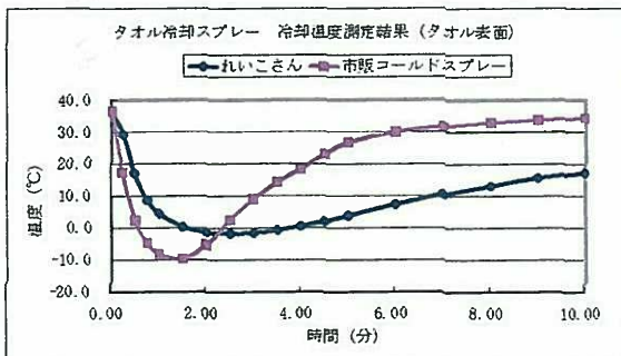
クールスプレー 冷却温度測定結果
